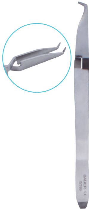
Pinza para colocar brackets con alineador. 11cm. Ref. 5/399
